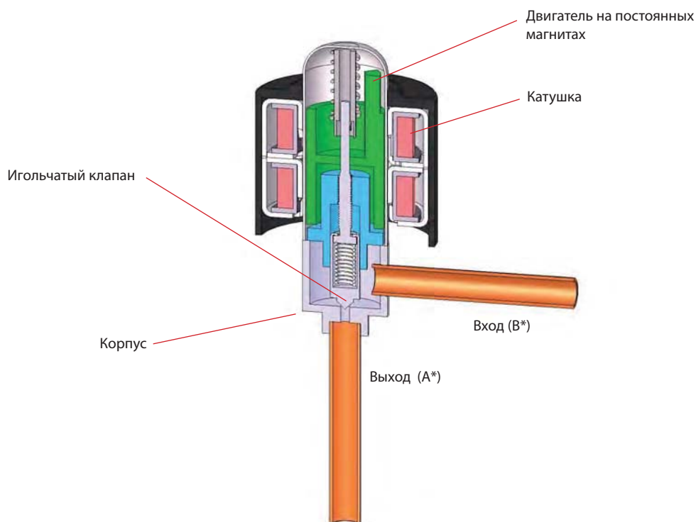
Чертеж поперечного сечения клапана серии ETS 6.
