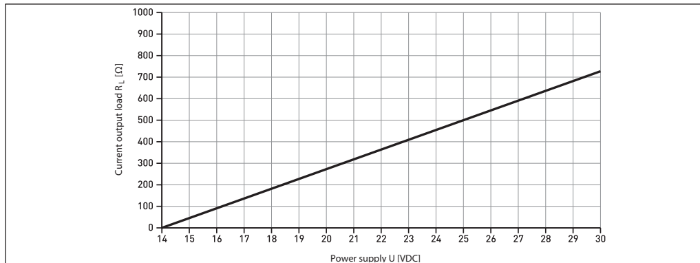
Минимальное значение питающего напряжения для выходного сигнала 22 мА
