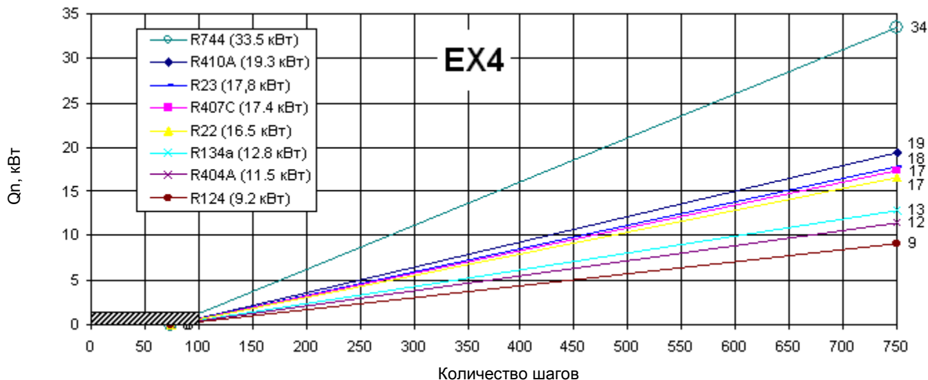
Диаграмма производительности (кВт)
